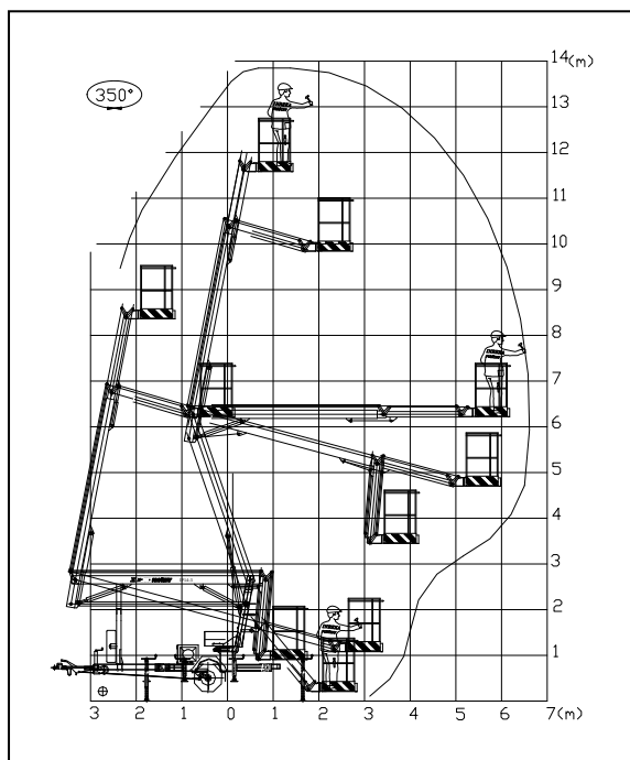
Pracovní diagram
